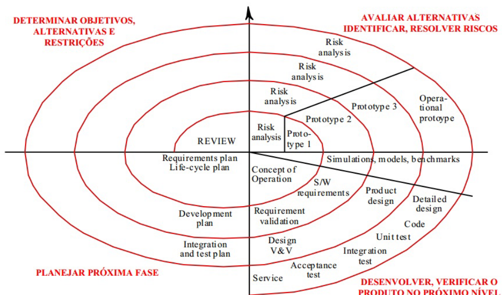
Figura 8 - Modelo Espiral.
