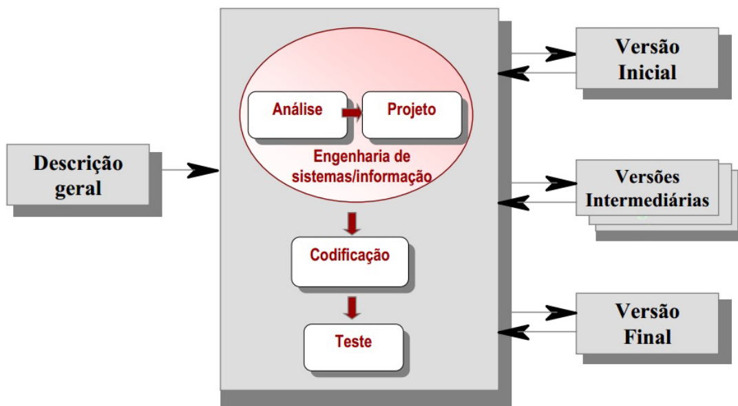
Figura 7- Modelo Incremental.
