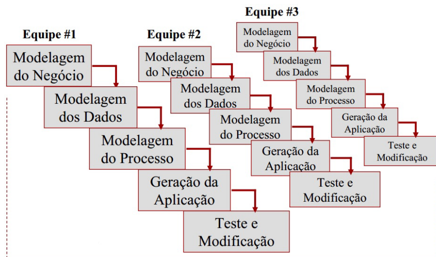
Figura 5 - Modelo RAD.
